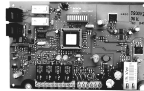
C900V2 → Dialer-Capture Ethernet Module
